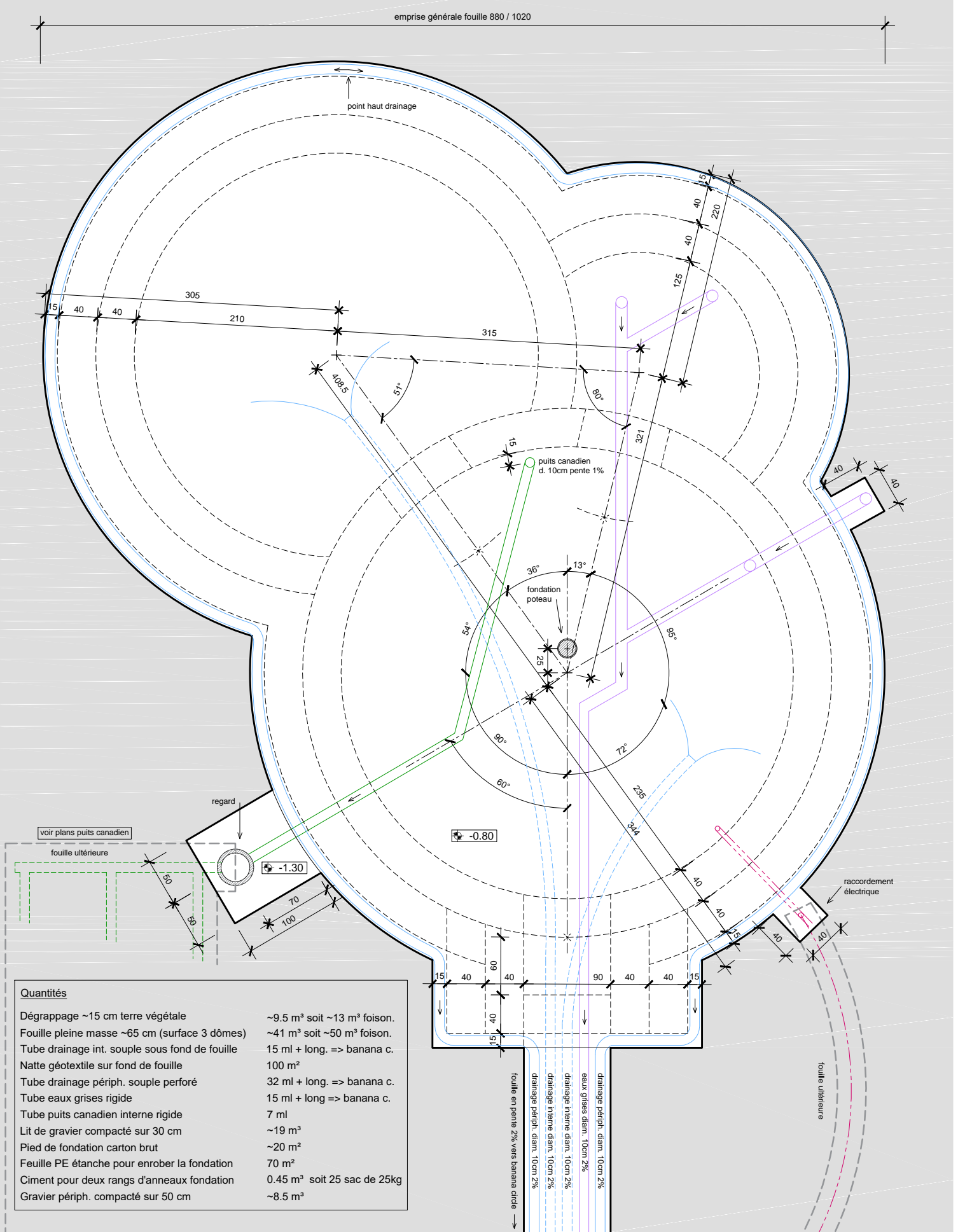
Plan fondation 1/50
