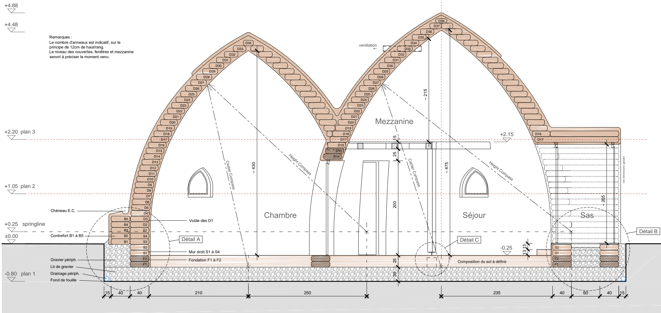
Coupe A - A 1/50
