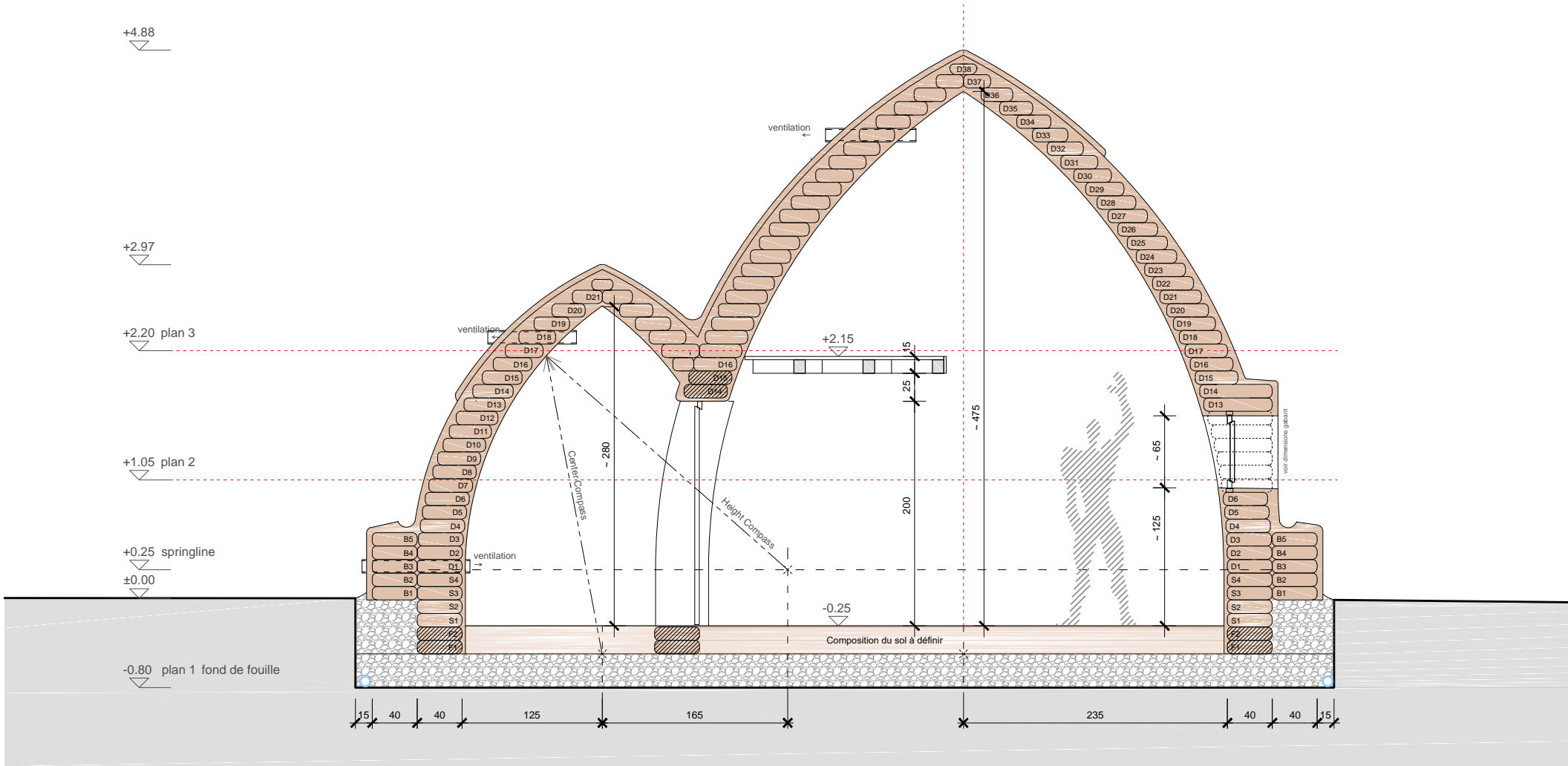
Coupe B - B 1/50
